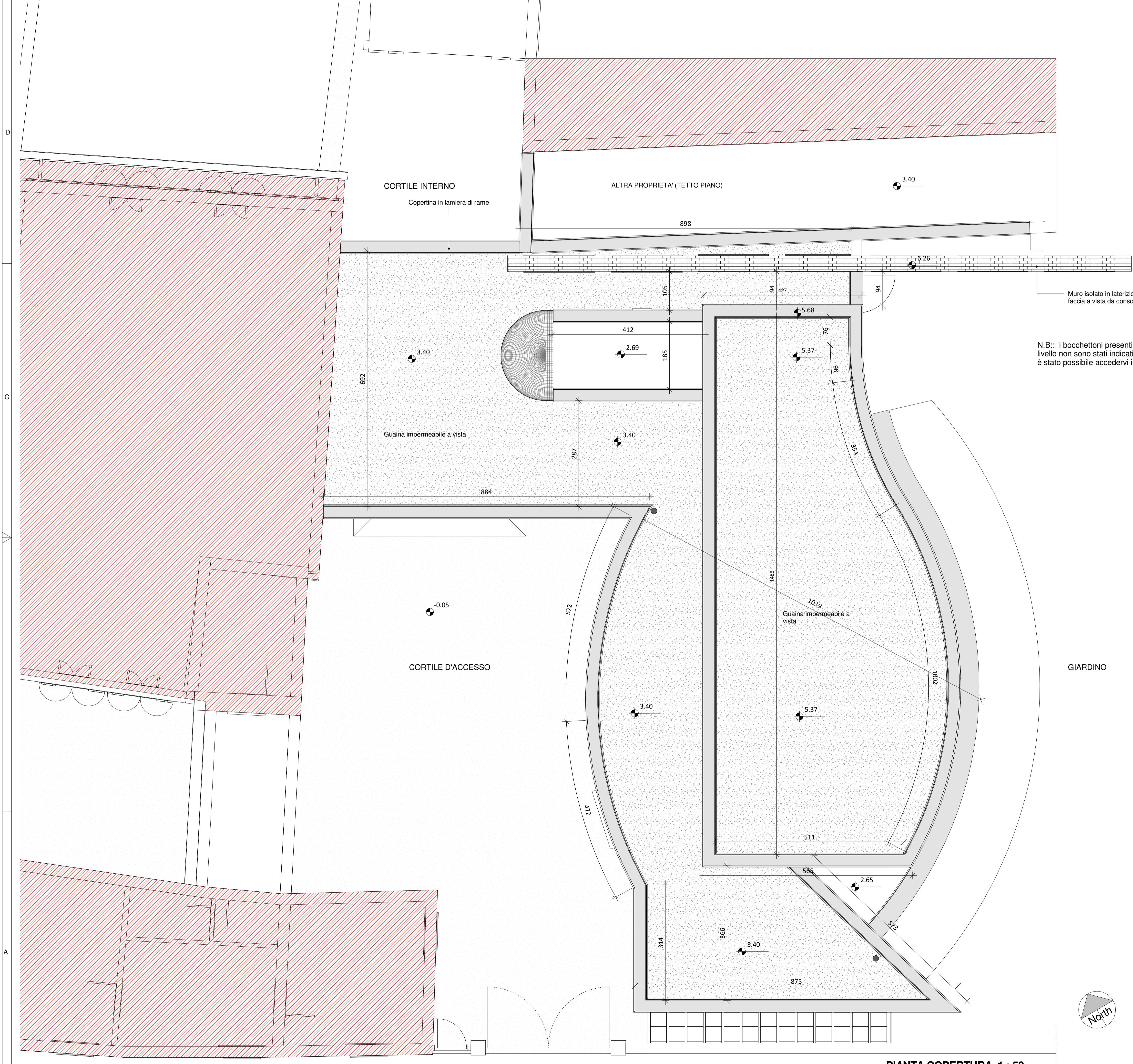
PIANTA COPERTURA 1 : 50
