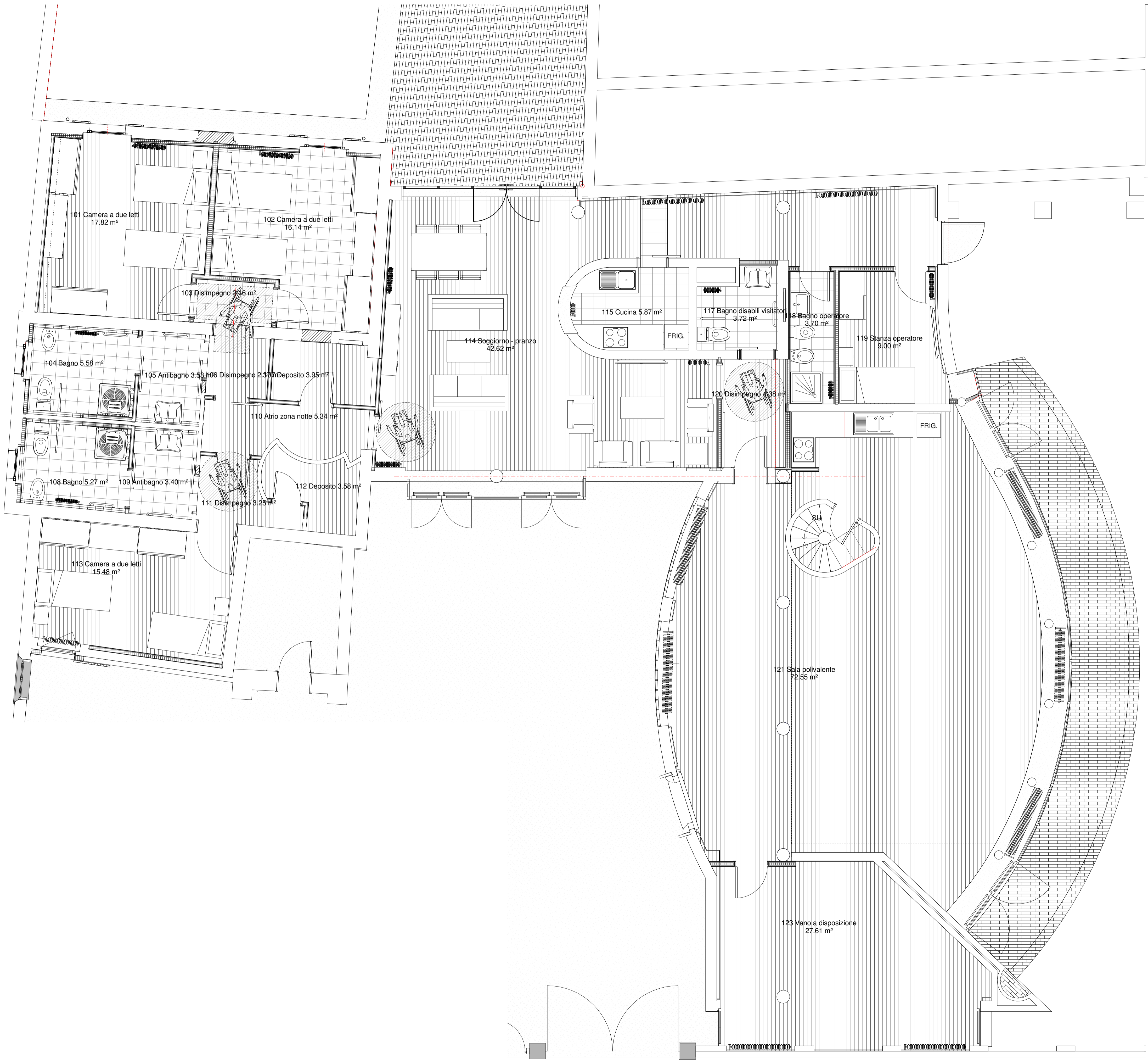
1 Pianta Arredi 1 : 50
